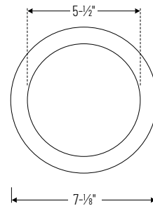
NELOCAC-6 6" ELO
