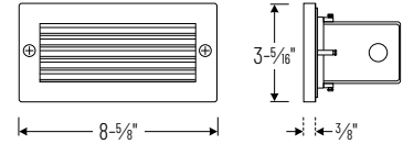
NSW-841/32 Louver
